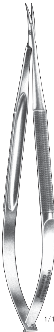
55 81 15 先端部： 形状/湾曲、刃長/10mm ハンドル部：径8mm 全 長：150mm
