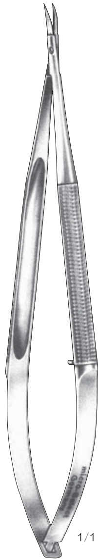
55 81 19 先端部(ヴァンナス型)： 形状/湾曲、刃長/5mm ハンドル部：径8mm 全 長：150mm
