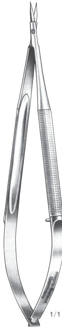
55 81 18 先端部(ヴァンナス型)： 形状/直、刃長/5mm ハンドル部：径8mm 全 長：150mm
